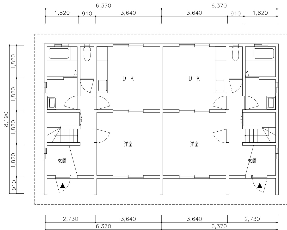
1 階 平 面 図
