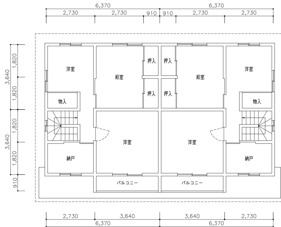
2 階 平 面 図
